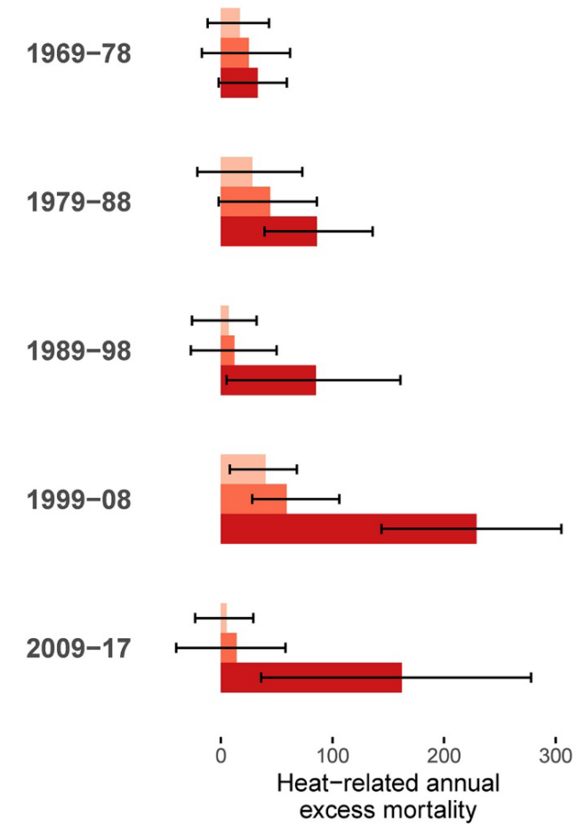
Hitzebedingte Sterblichkeit in der Schweiz
