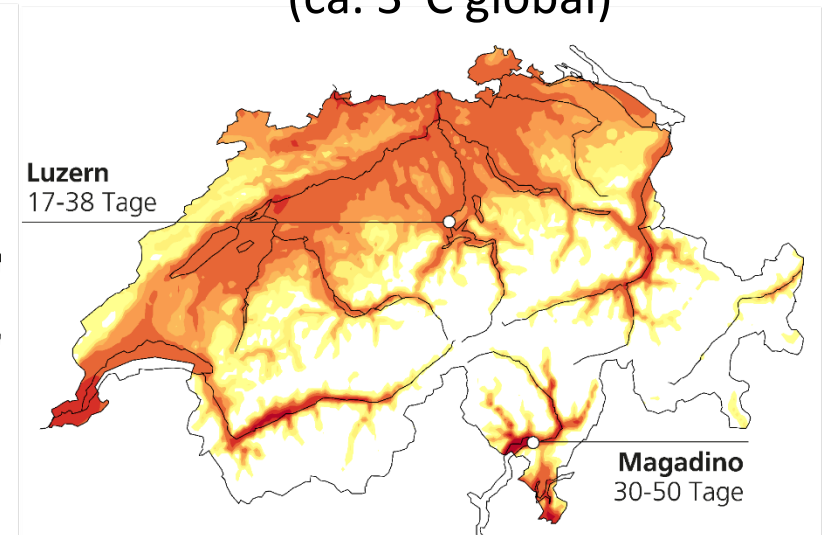
Ohne Klimaschutz 2060 (ca. 3°C global)
