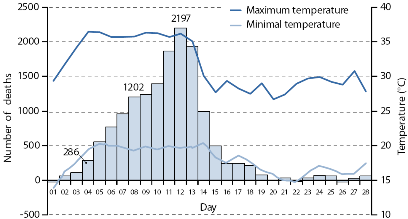
Übersterblichkeit in Frankreich 2003
