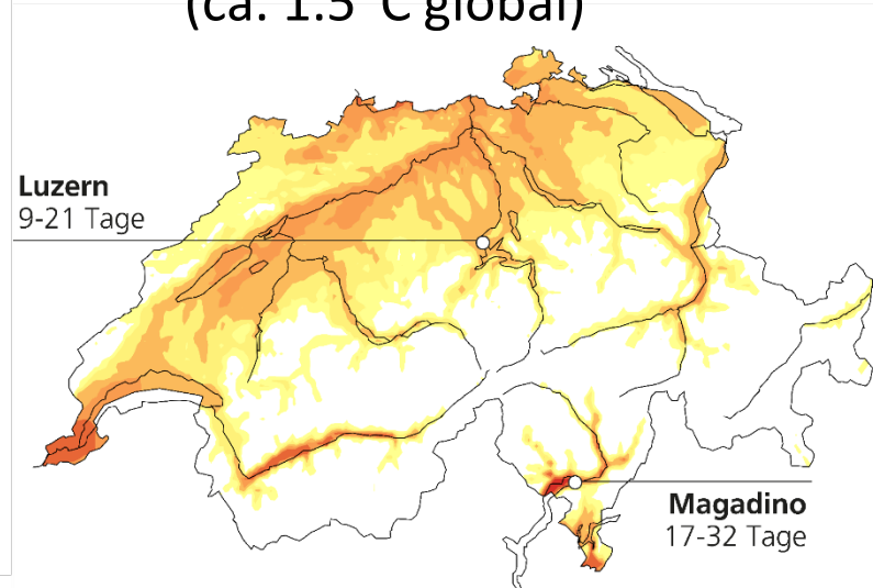
Konsequenter Klimaschutz 2060 (ca. 1.5°C global)
