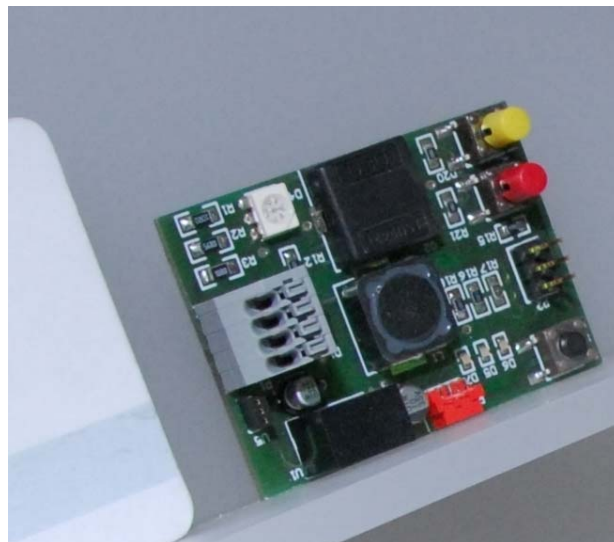
Bild 4a Lokalisierung mit Ultraschall: Empfänger
