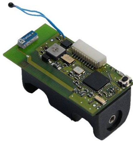
Bild 1 Der Sturzsensor iCare
