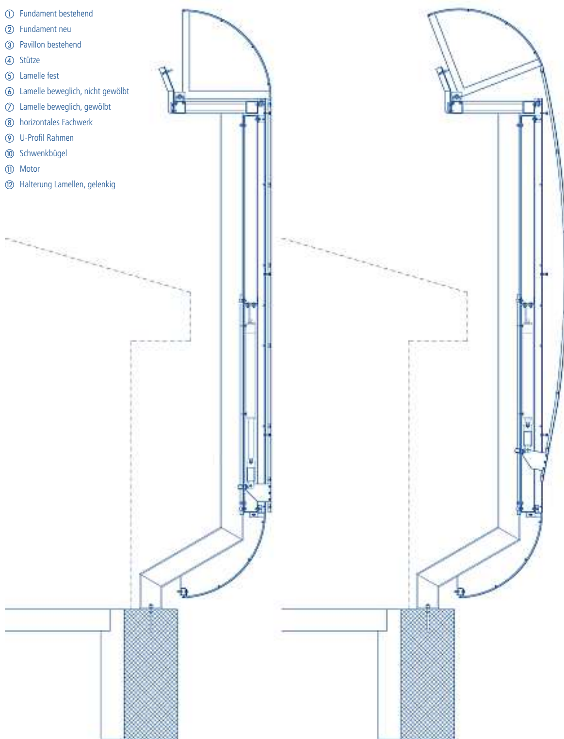
4 Vertikalschnitte Lamellen
