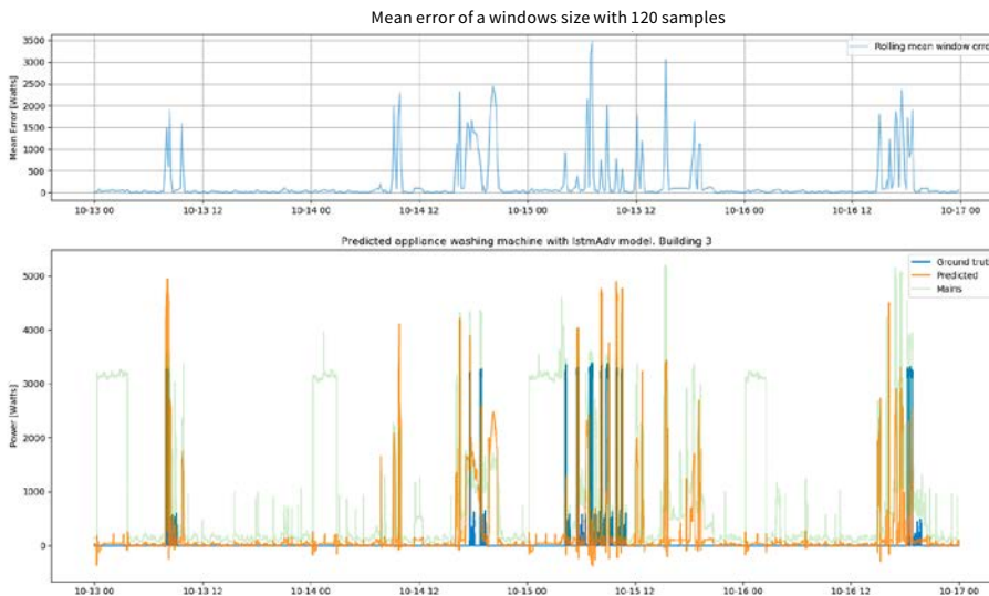
Die Grafik zeigt den gemessenen Lastgang einer Waschmaschine (Ground Truth in blau) sowie die mit der NIALM-Technologie erzeugte Verbrauchskurve (orange).
