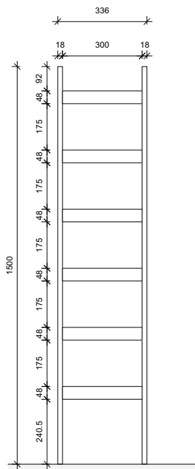
Ansicht frontal
