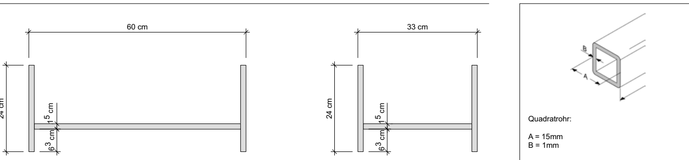
Ansichten Mst. 1:5
