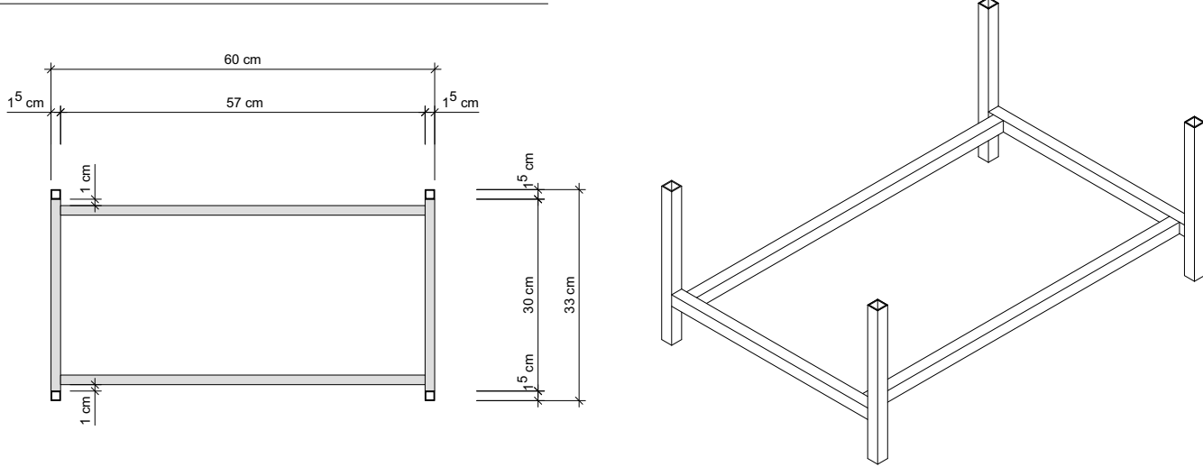
Grundriss Mst. 1:5
