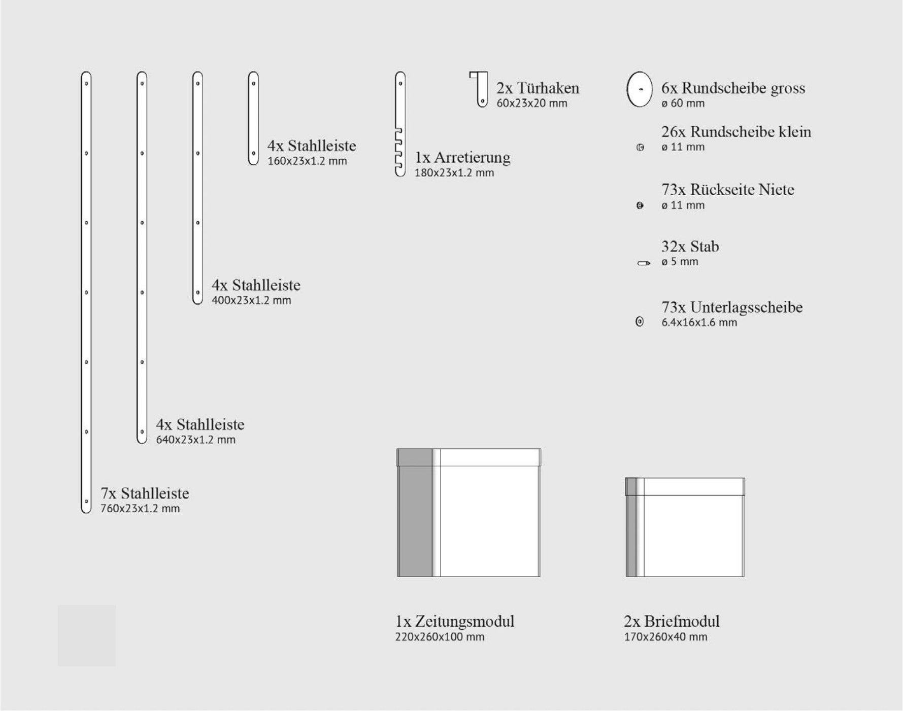
Stückliste vier Längen von Leisten | zusammengesetzt geliefert
