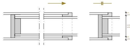
Ausziehbarer Rahmen | Stoppmechanismus mst.1:10
