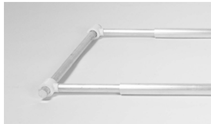
Rahmenprototyp 2 | Auszugsmechanismus
