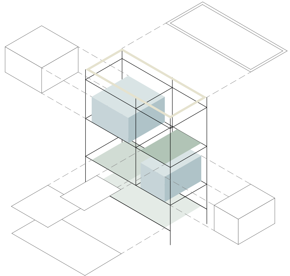
Herausnehmbare Elemente | Konstruktion agiert als Depot
