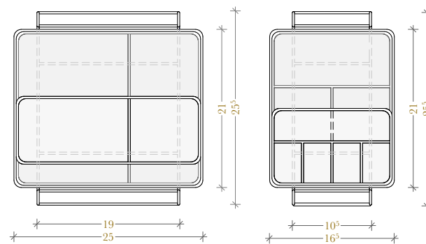
Boxen | Grundrisse & Ansichten im mst. 1:7
