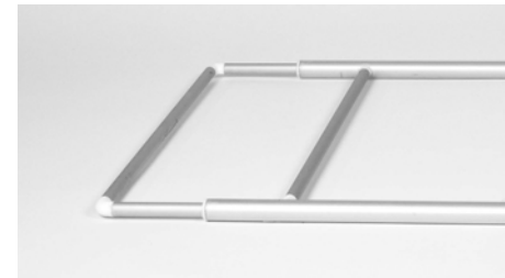
Rahmenprototyp 3 | Auszugsmechanismus
