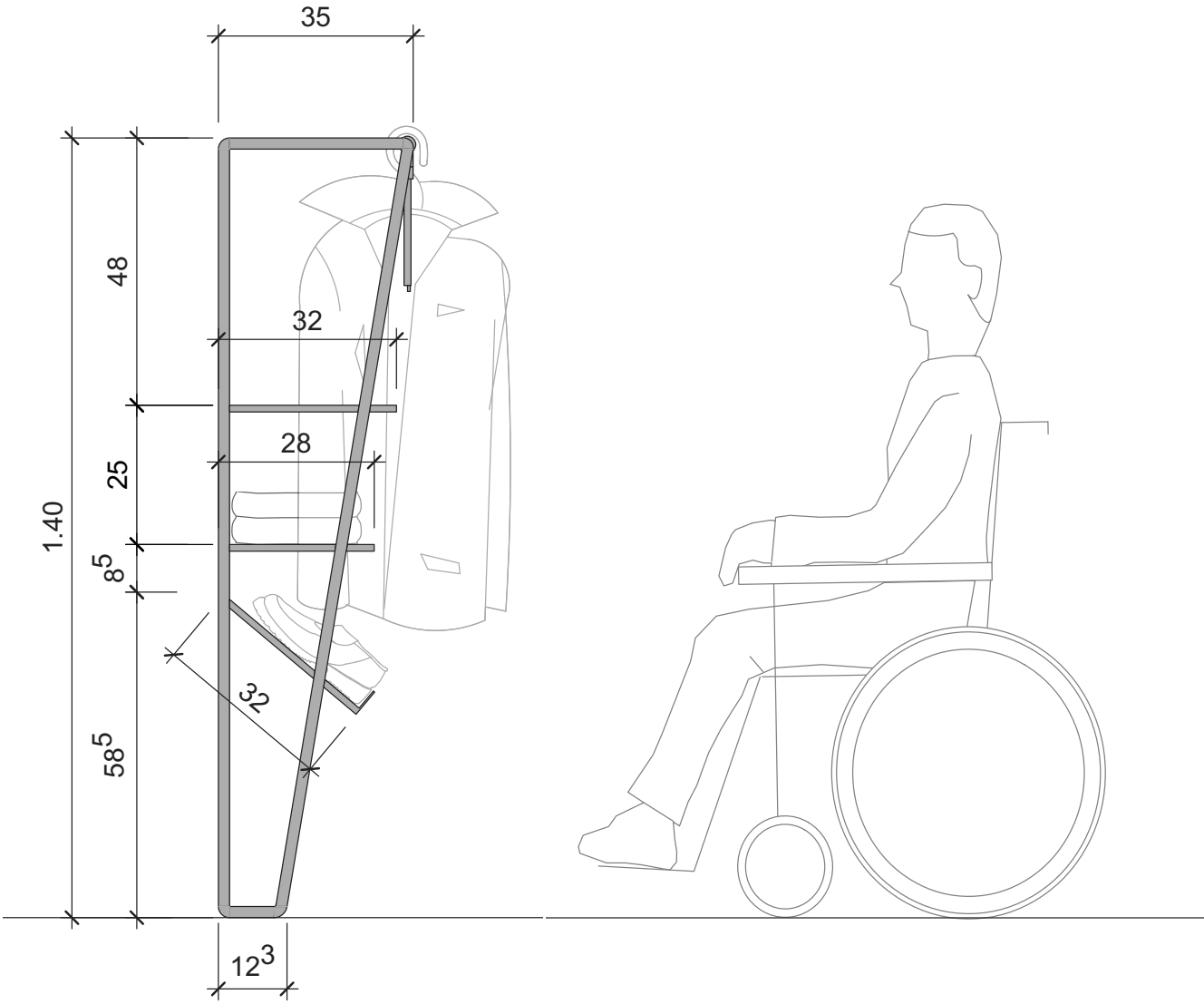
Seitenansicht Garderobe
