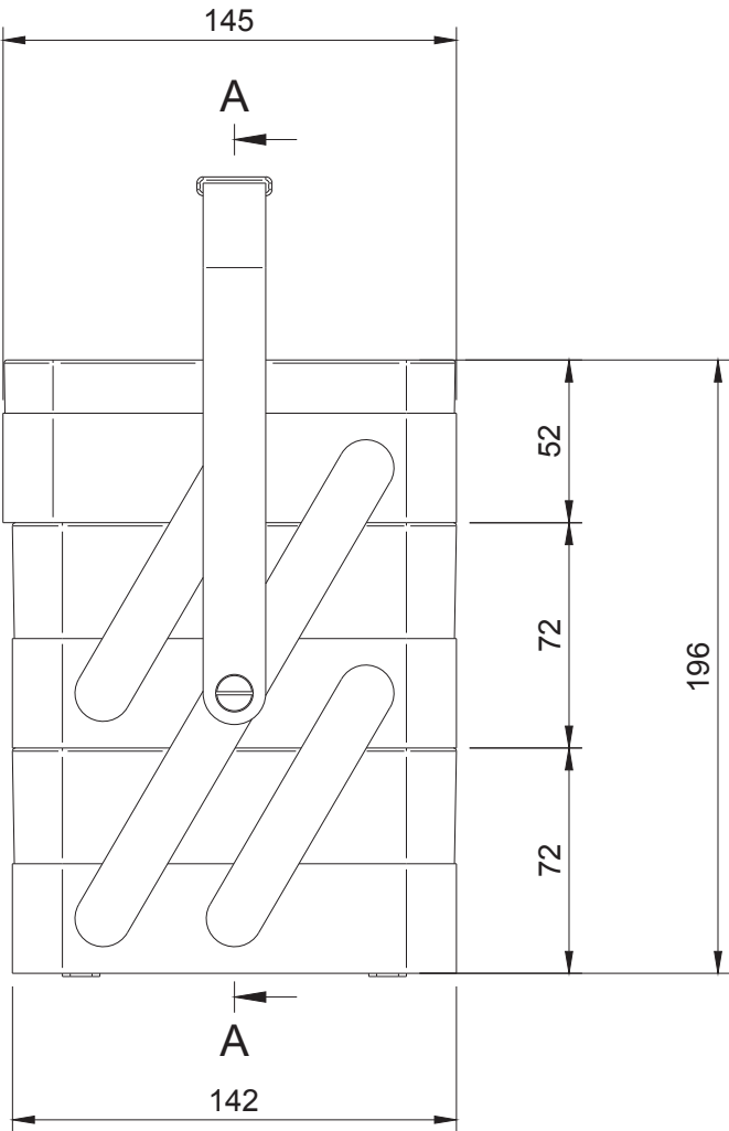
Anischt Seite MST 1:5
