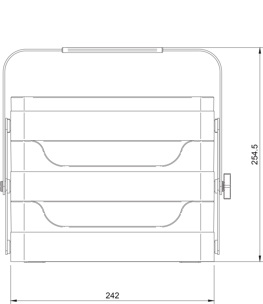
Ansicht Vorne MST 1:5
