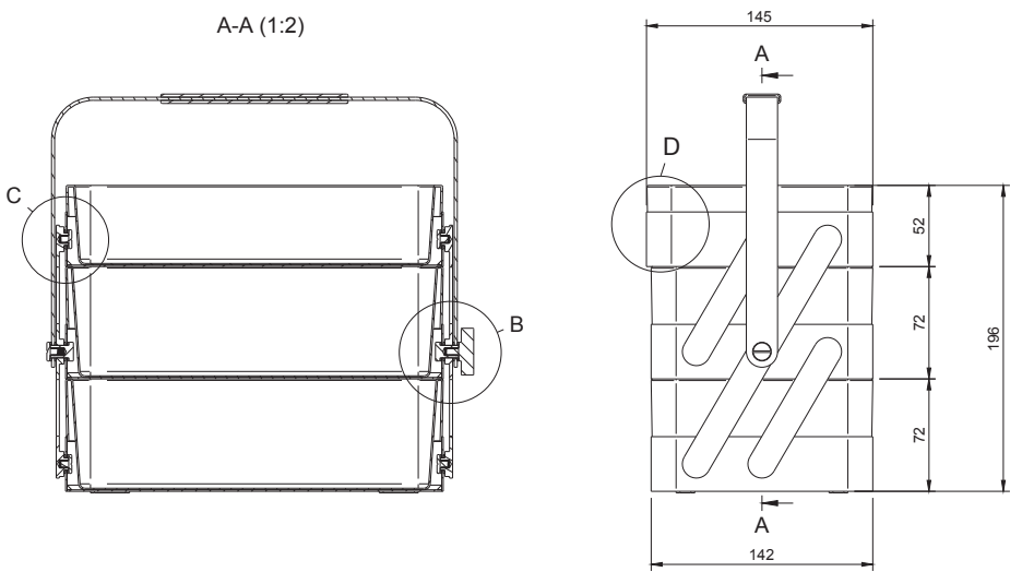
Schnitt A-A und Seiten Ansicht
