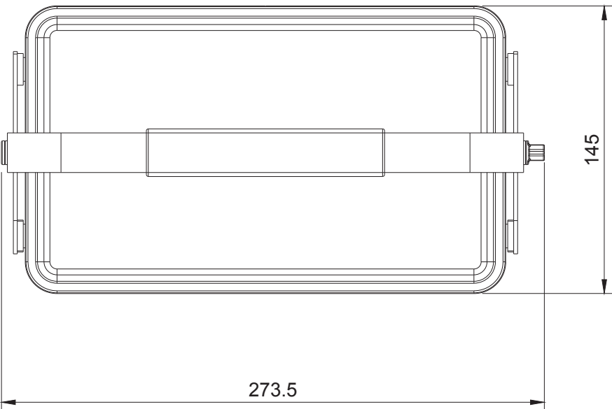
Draufsicht MST 1:5
