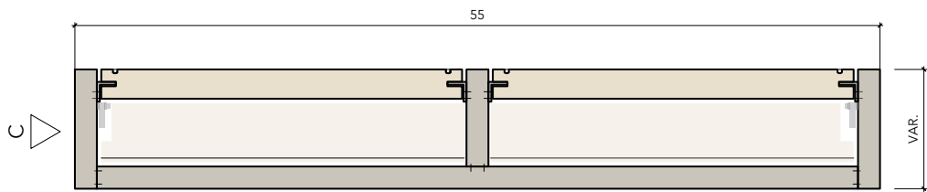
Längsschnitt B
