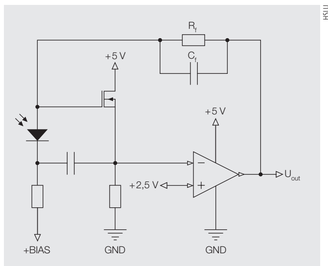
Bild 5 Schema Empfangsverstärker.
